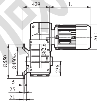
GFH/GFHZ/GFAF127输出轴
