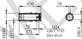
GFA/GFAZ/GFAF127输出轴
