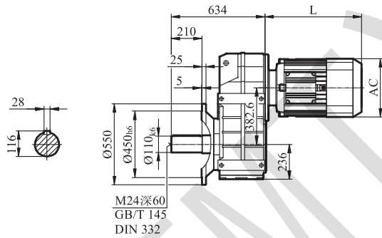
GFA/GFAZ/GFAF127输出轴
