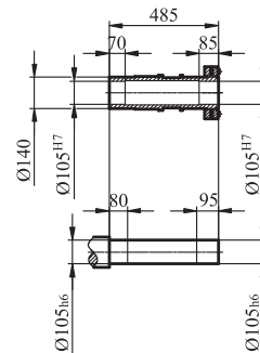
GFH/GFHZ/GFAF127输出轴
