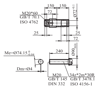
GKV/GKVZ/GKVF97输出轴
