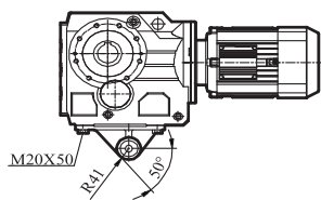
GKA/GKAZ/GKAF97输出轴
